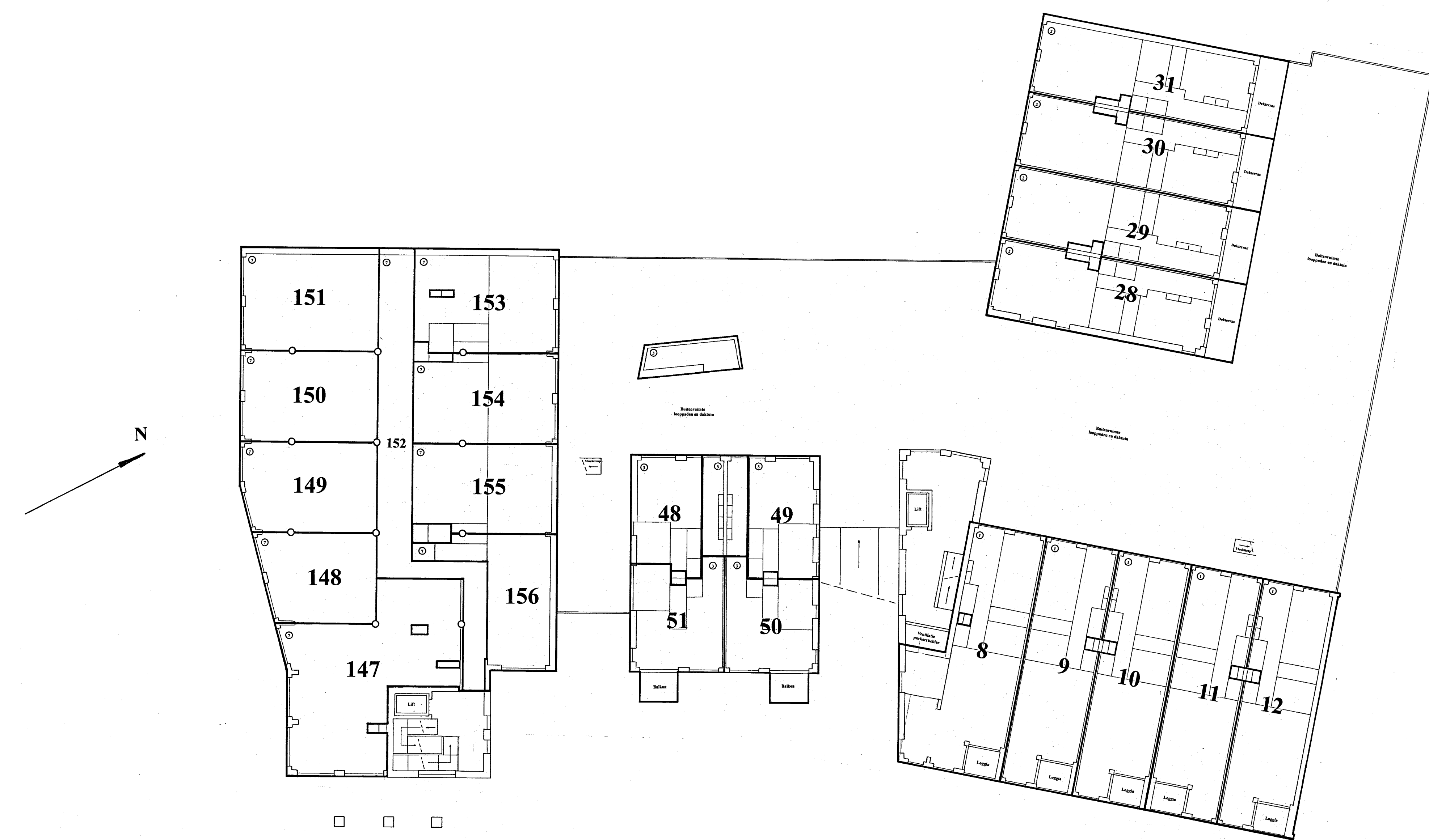
1e verdieping 1 : 200
