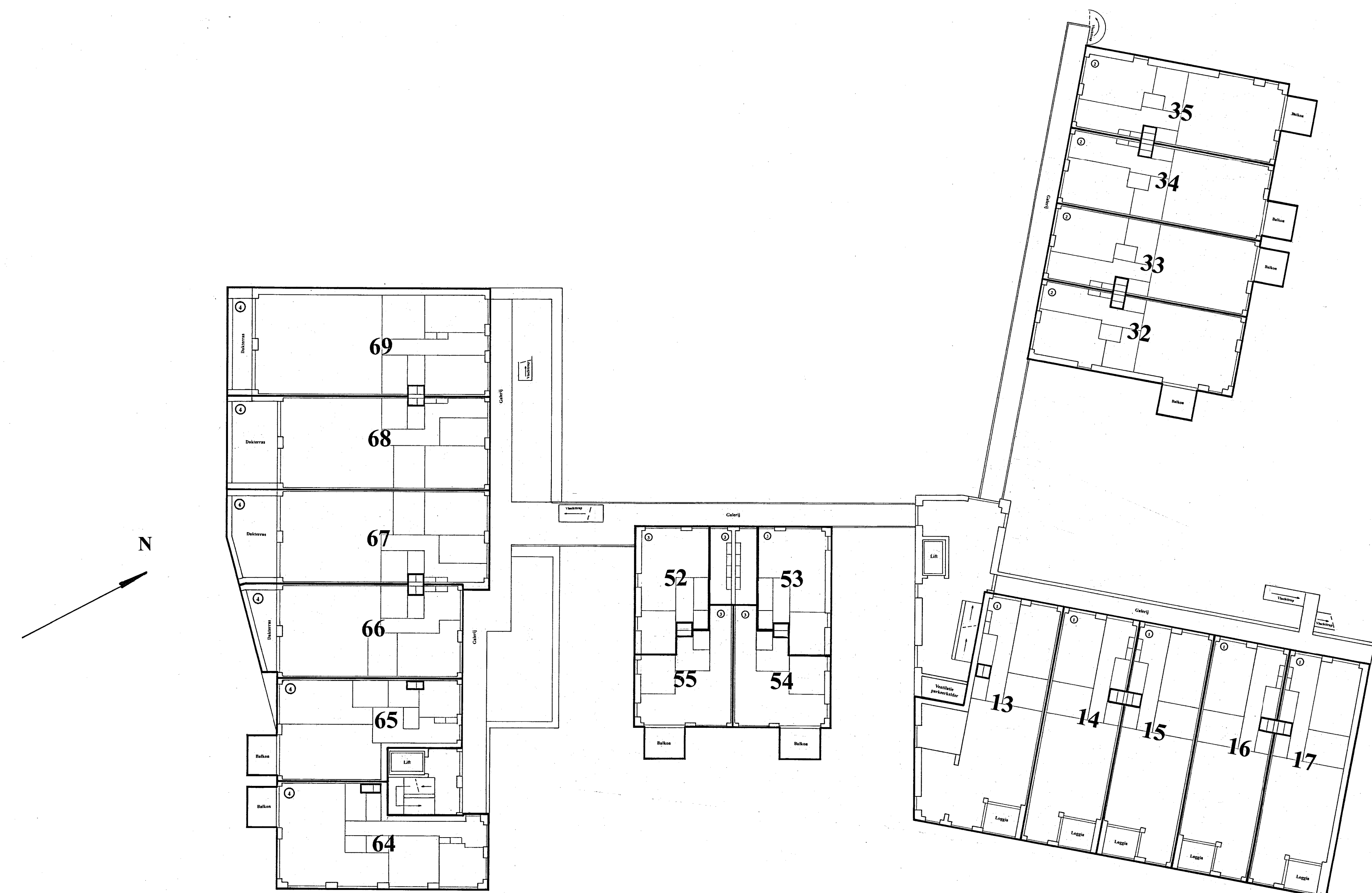
2e verdieping 1 : 200
