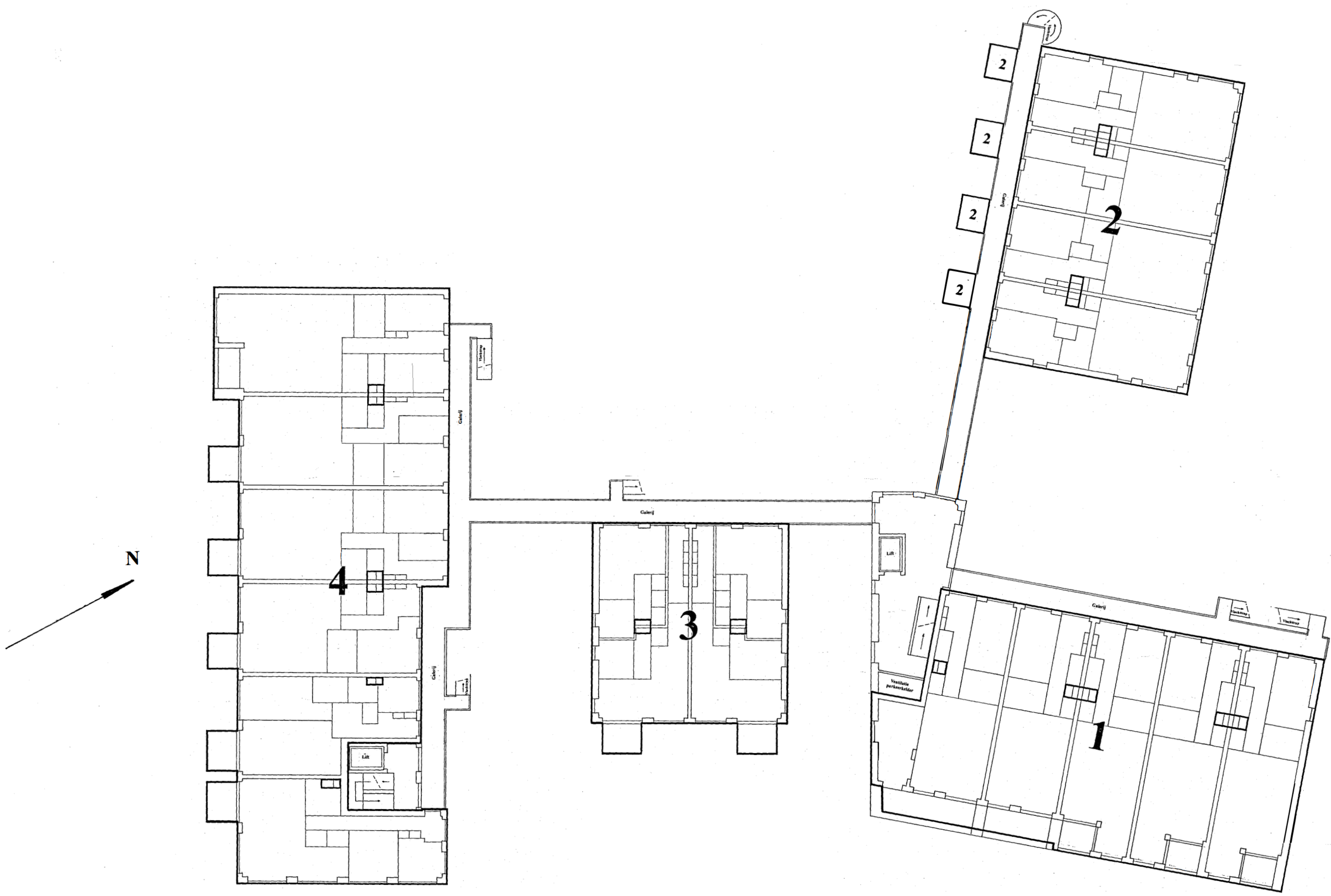
3 e verdieping 1 : 200
